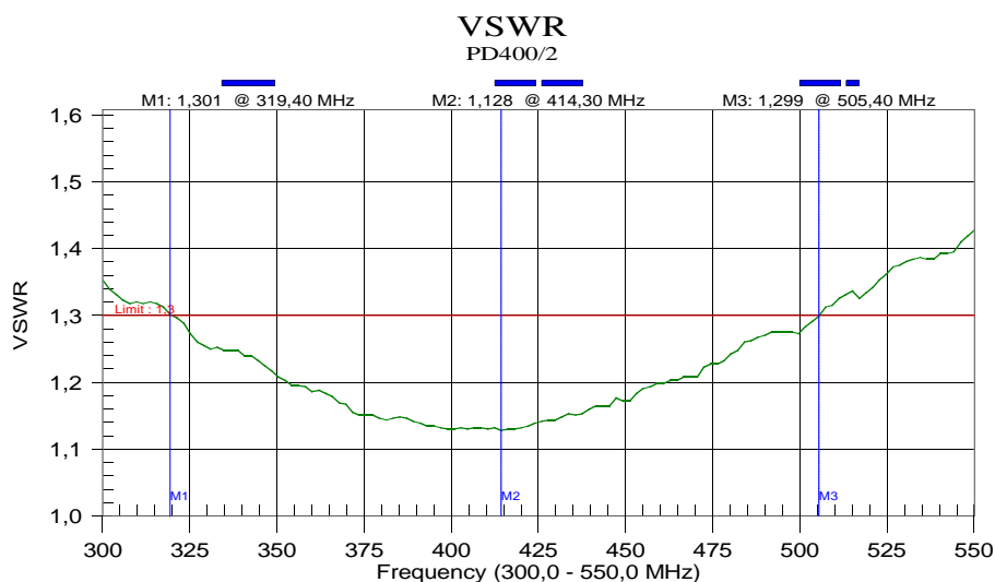
Przebieg charakterystyki VSWR dzielnika PD 400/2
