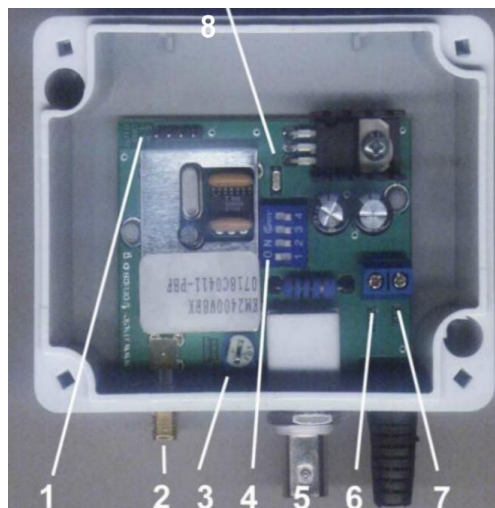
odbiornik VRX-2
