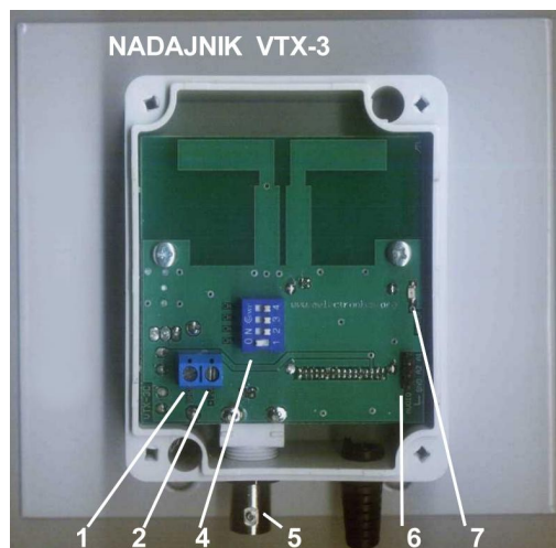
nadajnik VTX-3
