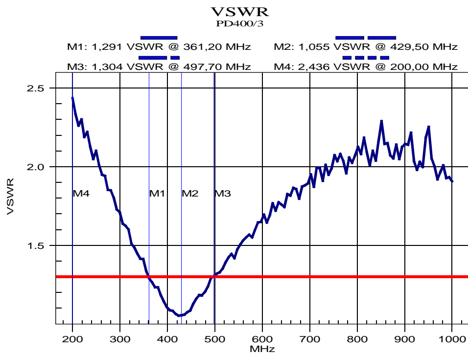
Przebieg charakterystyki VSWR dzielnika PD 400/3
